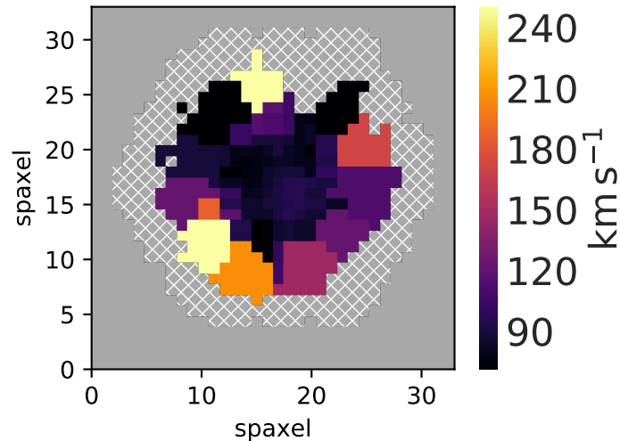
7443-12701 stellar_sigma
