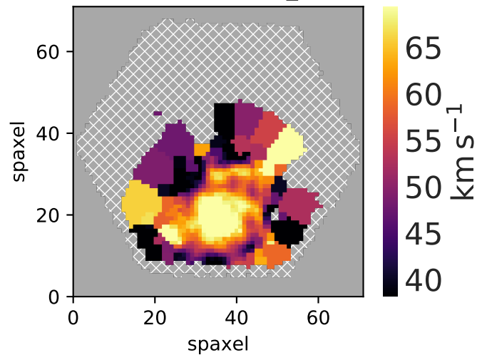
7443-12701 stellar_sigma
