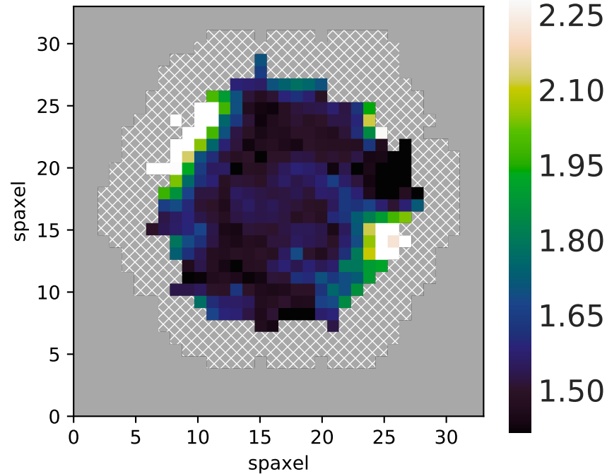
Spectral index: D4000
