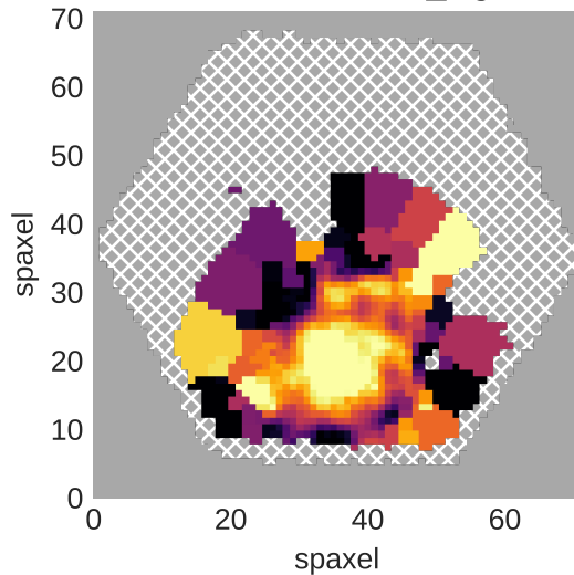
7443-12701 stellar_sigma
