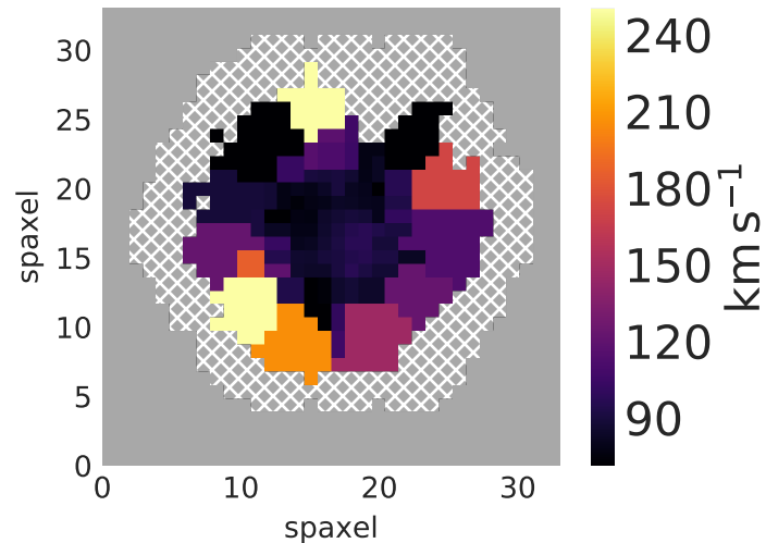
7443-12701 stellar_sigma
