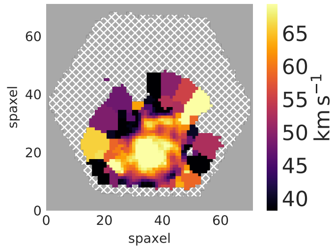
7443-12701 stellar_sigma
