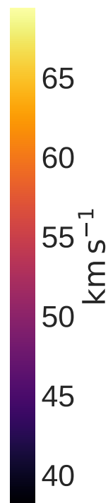
7443-12701 stellar_sigma
